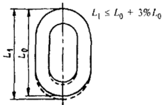
Рис. 1. Увеличение звена цепи:
