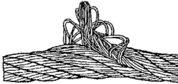
Рис. 11. Выдавливание сердечника
