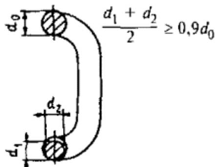
Рис. 2. Уменьшение диаметра сечения звена цепи:
