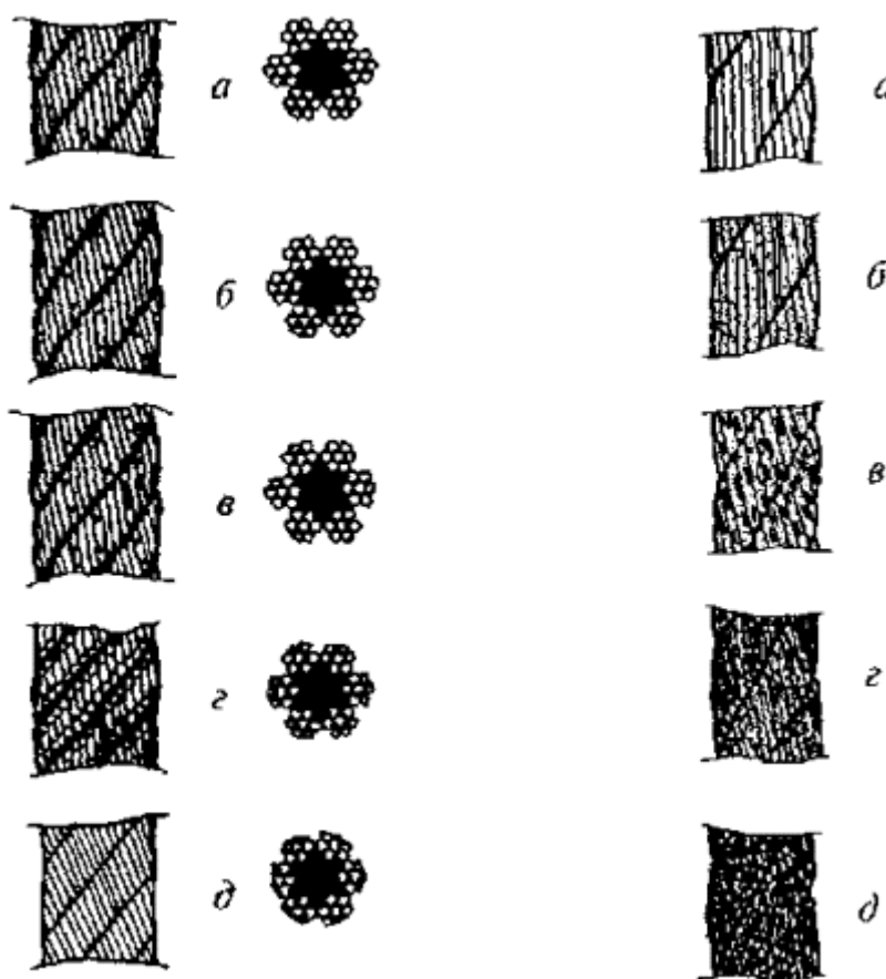
Рис. 5. Износ наружных проволок каната крестовой свивки:
