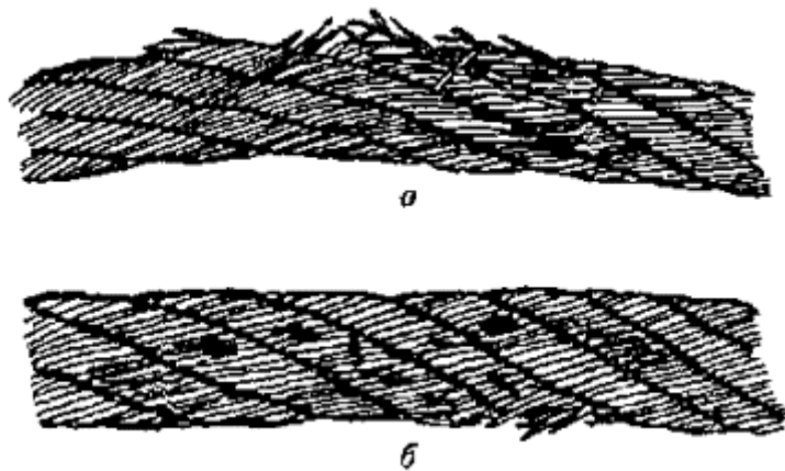
Рис. 3. Обрывы проволок в зоне уравнильного блока:
