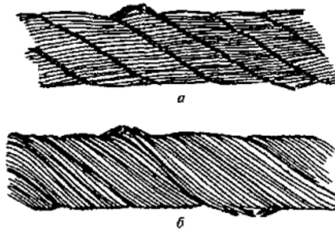
Рис. 2. Сочетание обрывов проволок с их износом:
